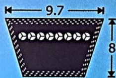
SECTION SPZ
