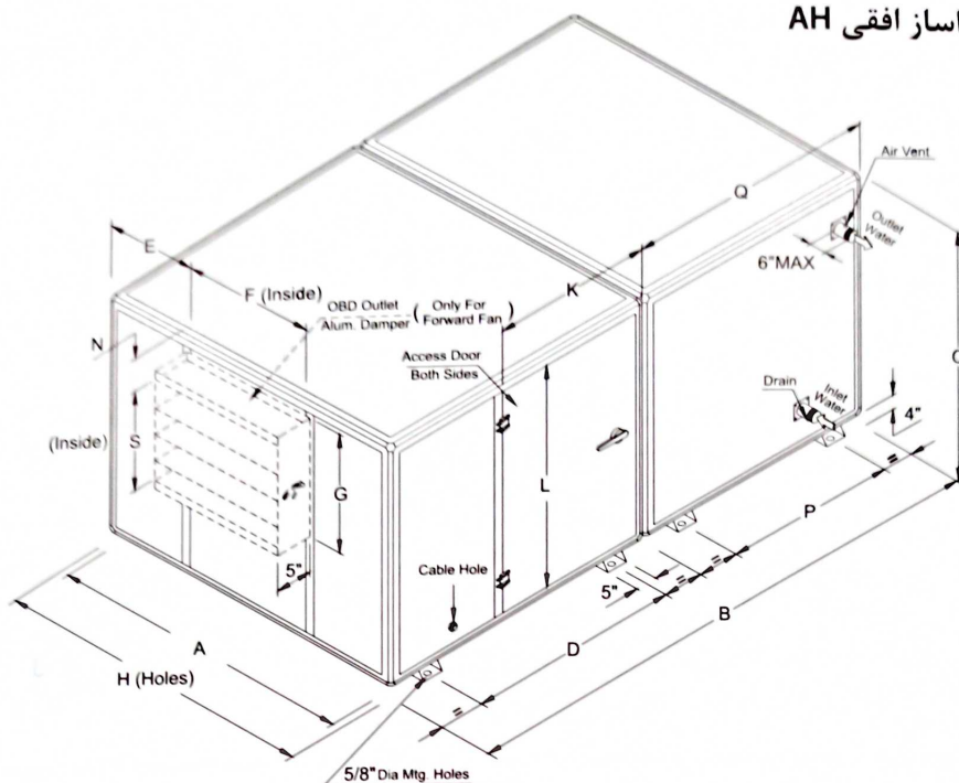
جدول ۴۸: مشخصات ابعادی هواساز افقی AH
