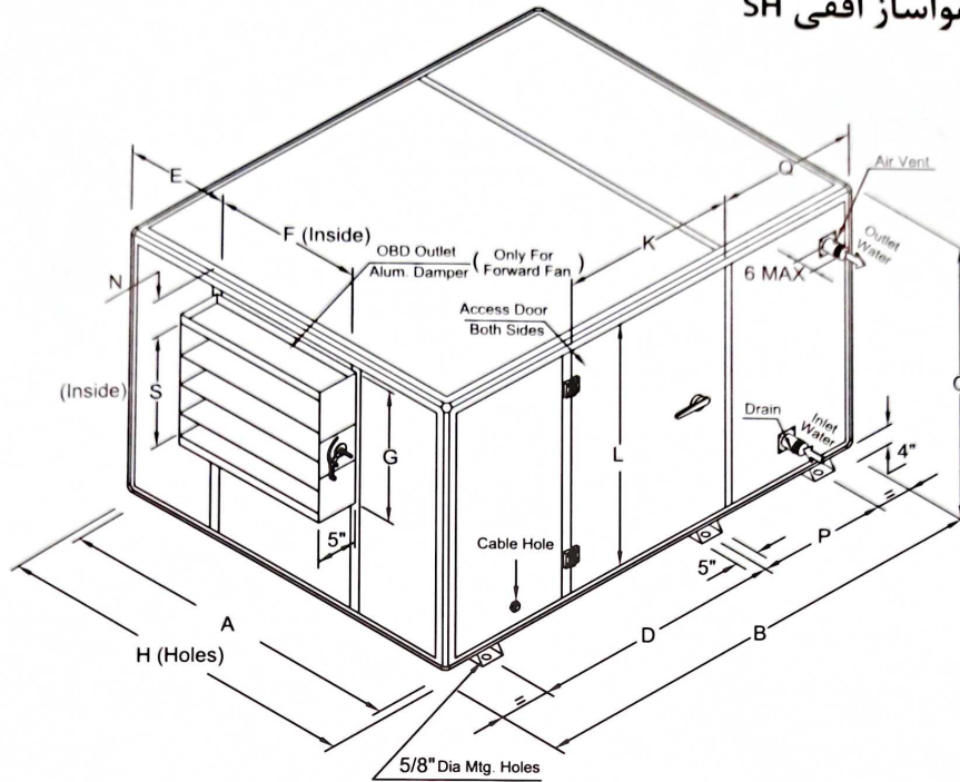
جدول ۴۷: مشخصات ابعادی هواسازهای افقی SH
