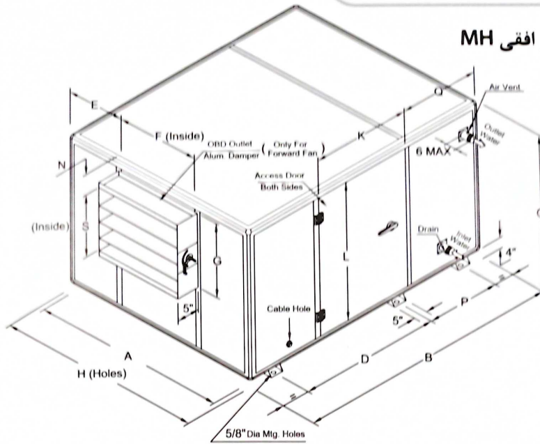
جدول ۴۹: مشخصات ابعادی هواساز افقی MH
