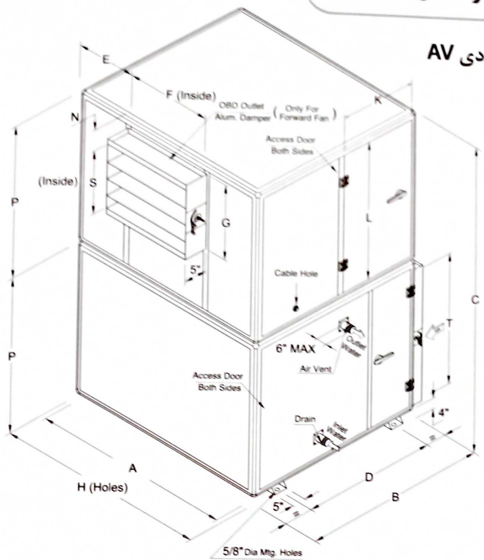
جدول ۵۱: مشخصات ابعادی هواساز عمودی AV
